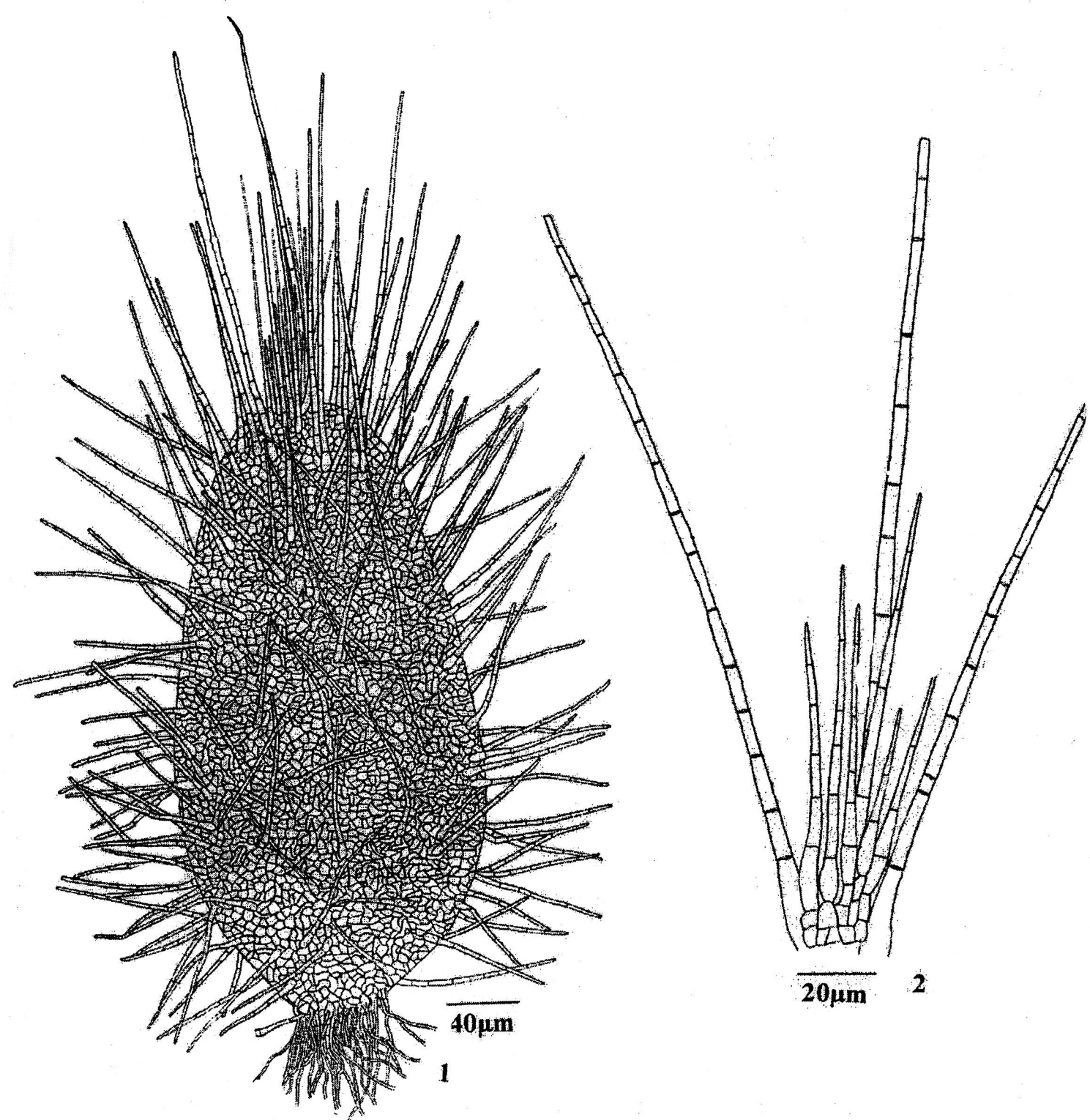
Chaetomium sp. - 5-1 (菌株 11272) 1. 子囊果, 2. 子囊果顶部孔口的局部结构 (内侧观, 示孔口毛特征)
