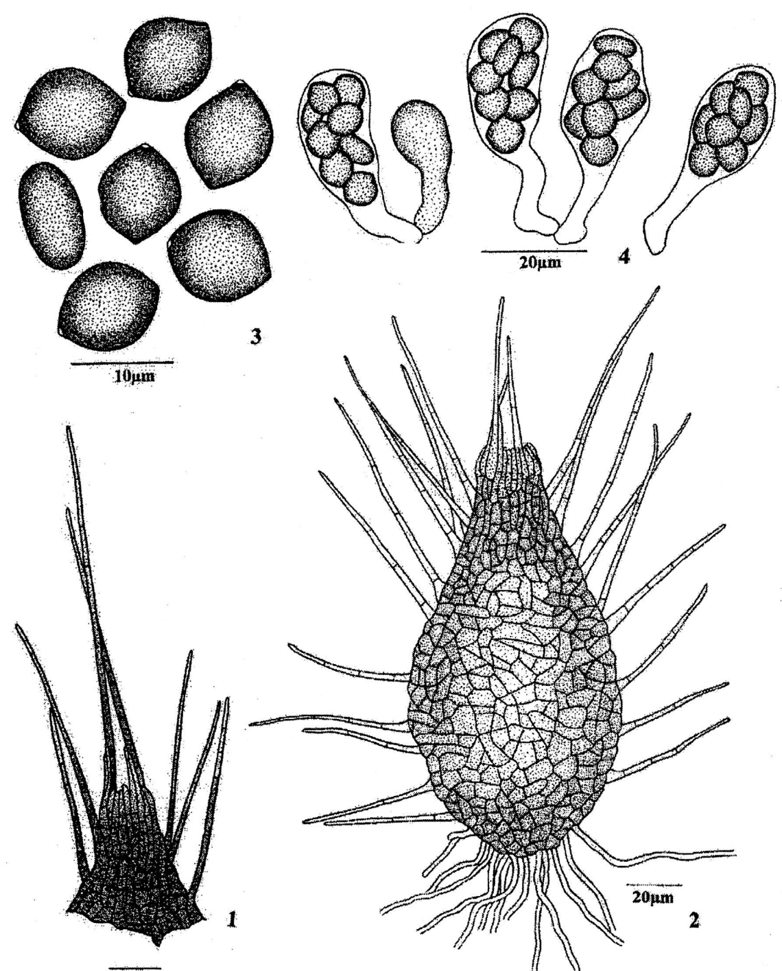
C. seminudum 1. 子囊果顶部结构 (示退化的孔口毛), 2. 子囊果, 3. 子囊孢子, 4. 子囊
