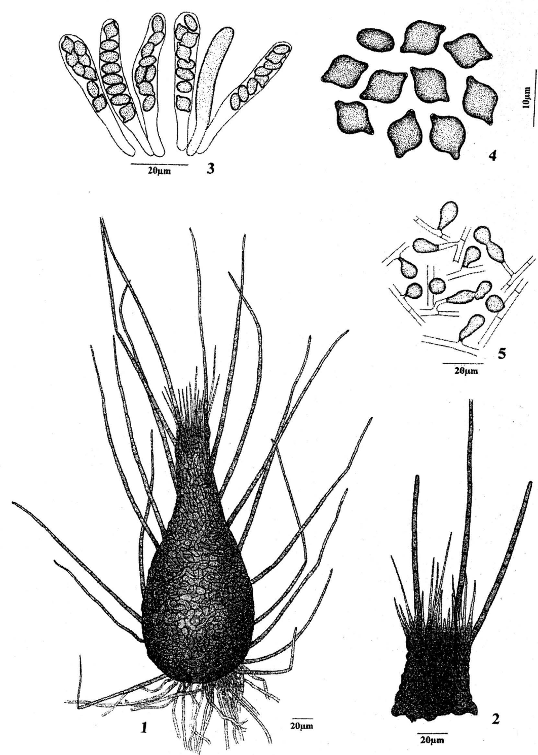
Chaetomium sp. nov. - 2 1. 子囊果, 2. 子囊果顶部结构 (示孔口毛特征), 3. 子囊, 4. 子囊孢子, 5. 侧生厚垣孢子
