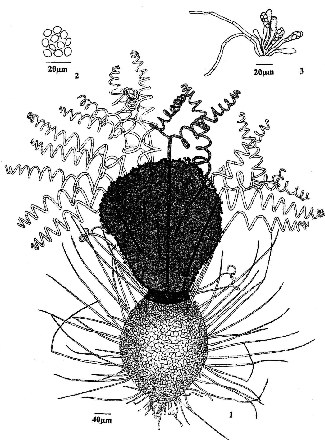
C. bostrychodes 1. 子囊果, 2. 子囊孢子, 3. 子囊束及侧丝
