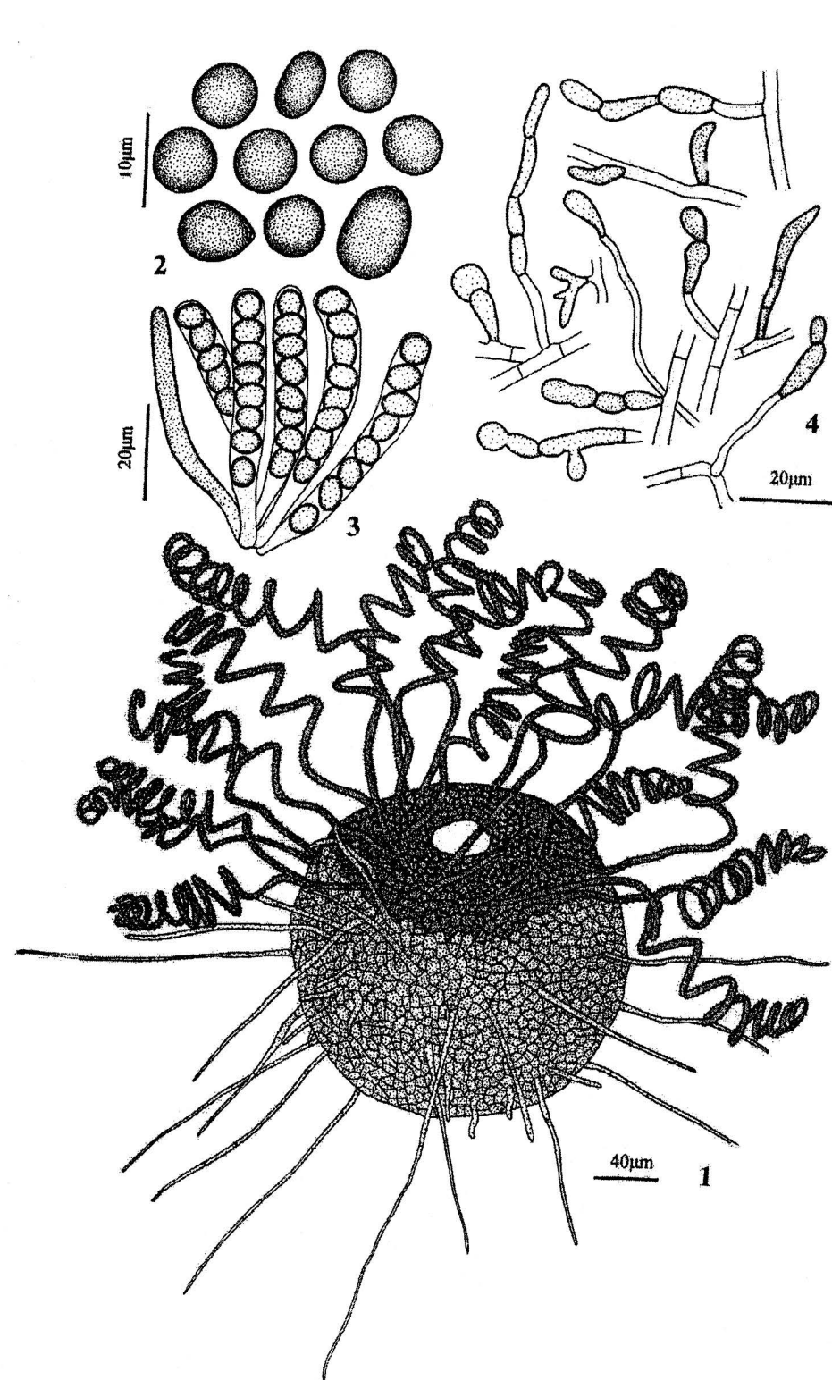
Chaetomium sp. nov. - 1 1. 子囊果, 2. 子囊孢子, 3. 子囊, 4. 厚垣孢子
