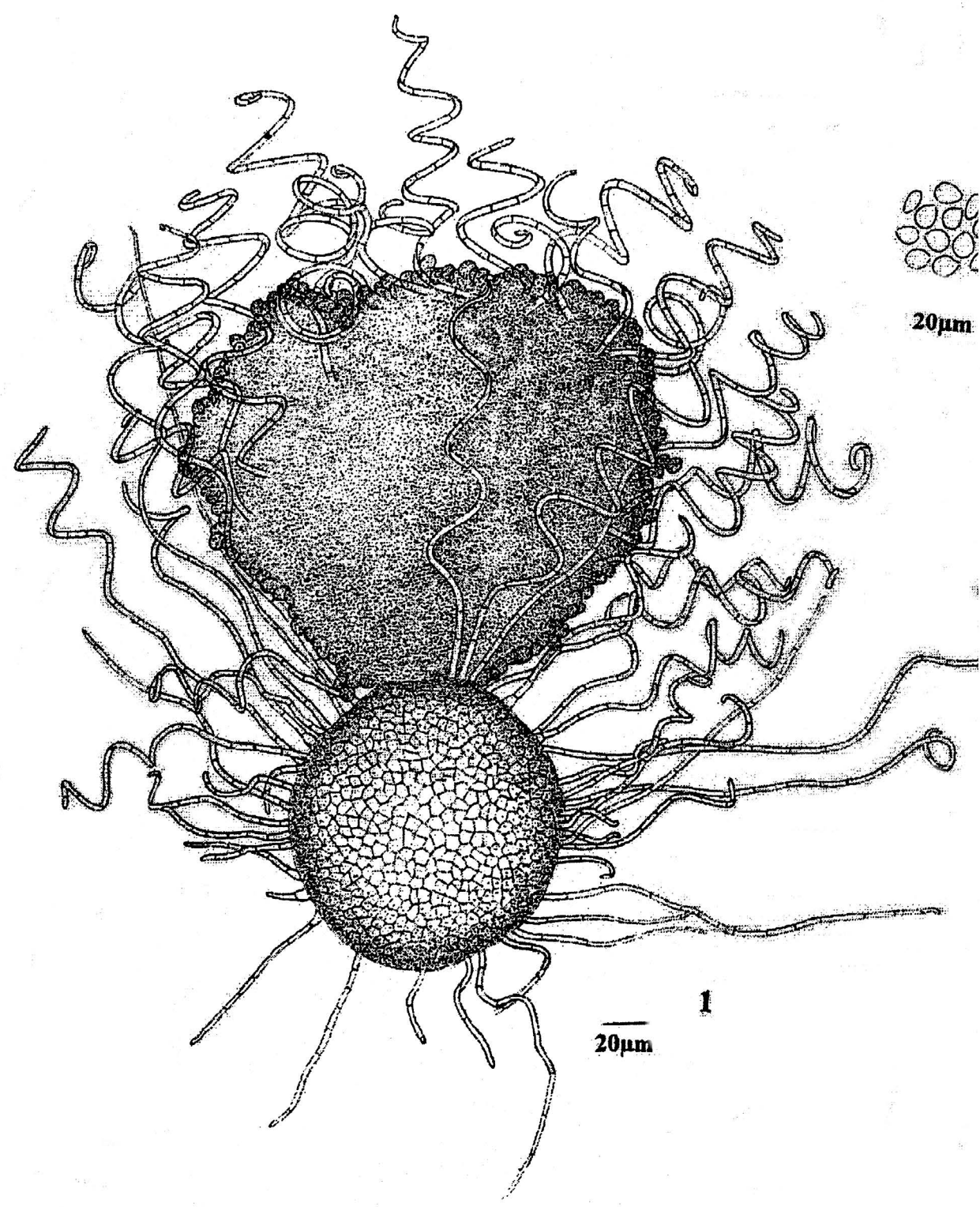
C. brasiliense 1. 子囊果, 2. 子囊孢子
