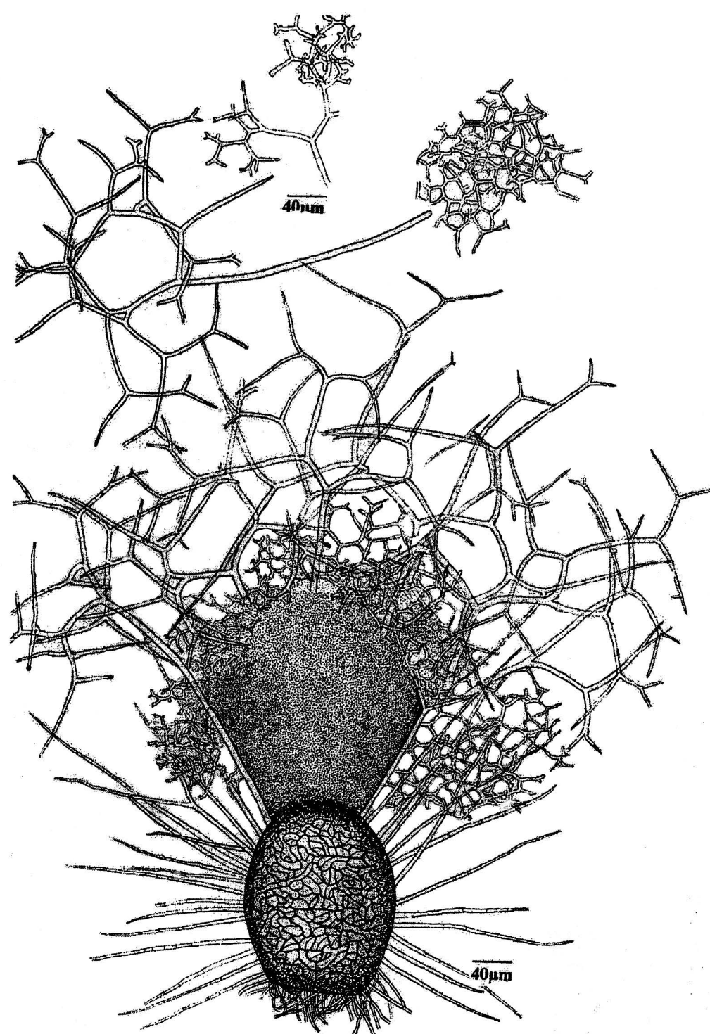
C. indicum 示子囊果及其顶生毛特征 (绘自菌株 8444)
