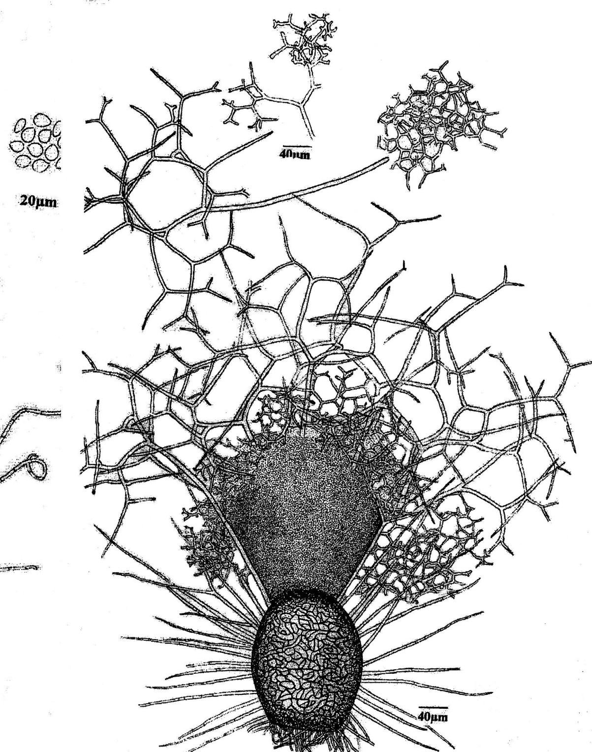
C. indicum 示子囊果及其顶生毛特征 (绘自菌株 8444)
